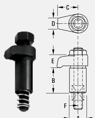
Stud and Nut Style
